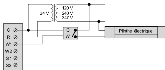
Plinthe électrique
