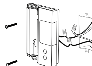
Installation à 4 fils
