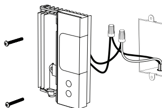
Installation à 2 fils
